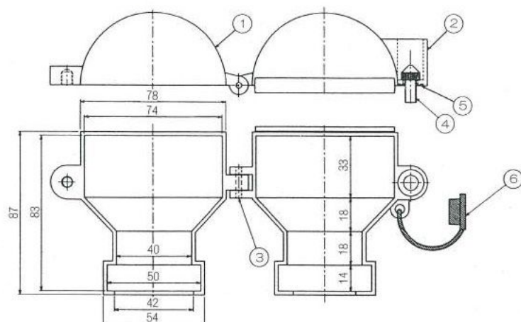
●閉栓キャップ〔M・S型〕
