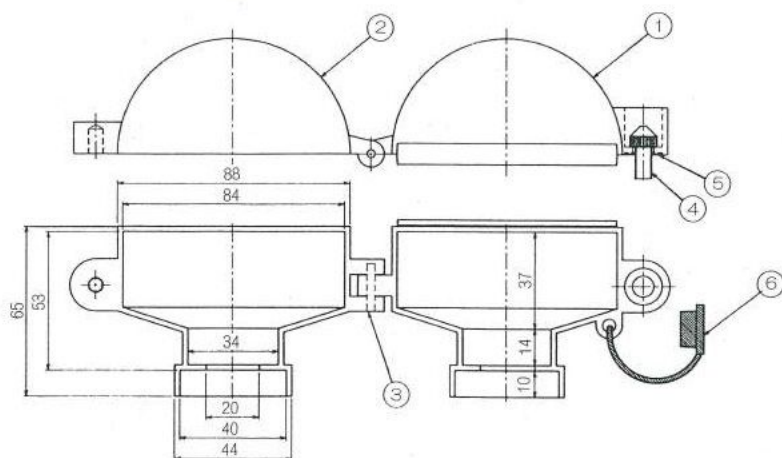
●閉栓キャップ〔L型〕
