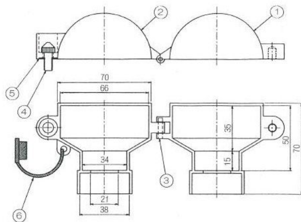
●閉栓キャップ〔S型〕
