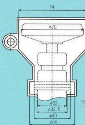
MS型 20mm×13mm兼用停水キャップ
