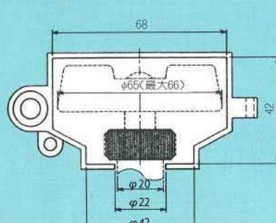
25mm 20mm ボール止水栓(ハンドル金属製)
