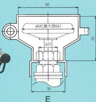
S型 13mm 丸ハンドル止水栓用
