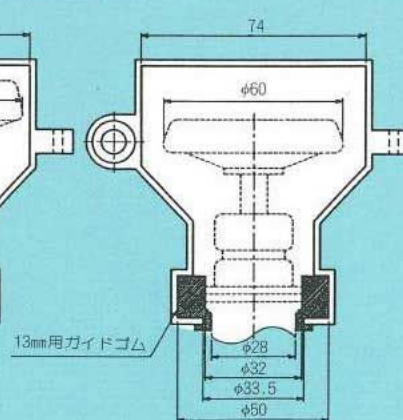
MS型 20mm×13mm兼用停水キャップ
