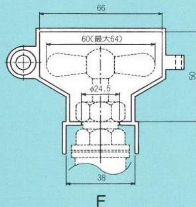
S型 20mm トンボハンドル止水栓用
