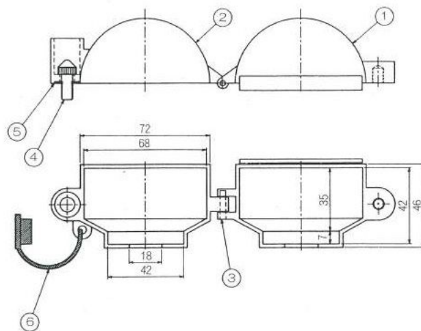
●閉栓キャップ〔S-II型〕
